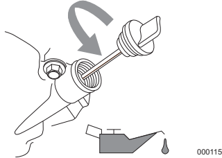
Figura 2-9. Sacar la varilla
