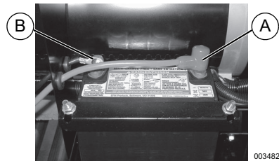
Figure 2-13. Raccorder la batterie
